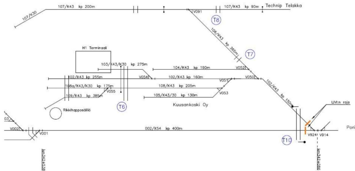
Porin sataman raiteistokaavio: Kirri (itäinen osa).
