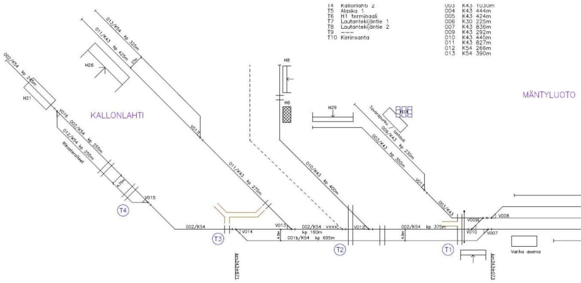
Porin sataman raiteistokaavio: Kallonlahti (länsiosa).
