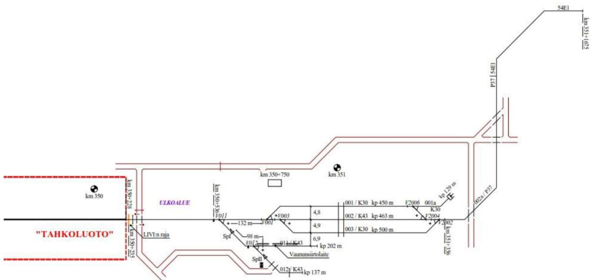
Porin sataman raiteistokaavio: Tahkoluoto.
