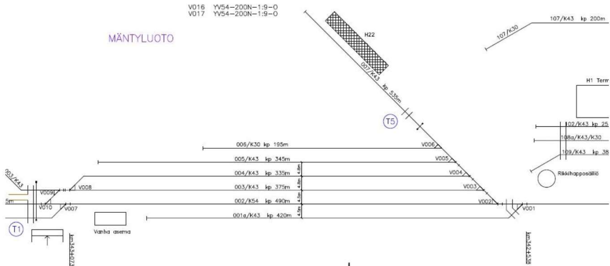
Porin sataman raiteistokaavio: Mäntyluoto (keskiosa).
